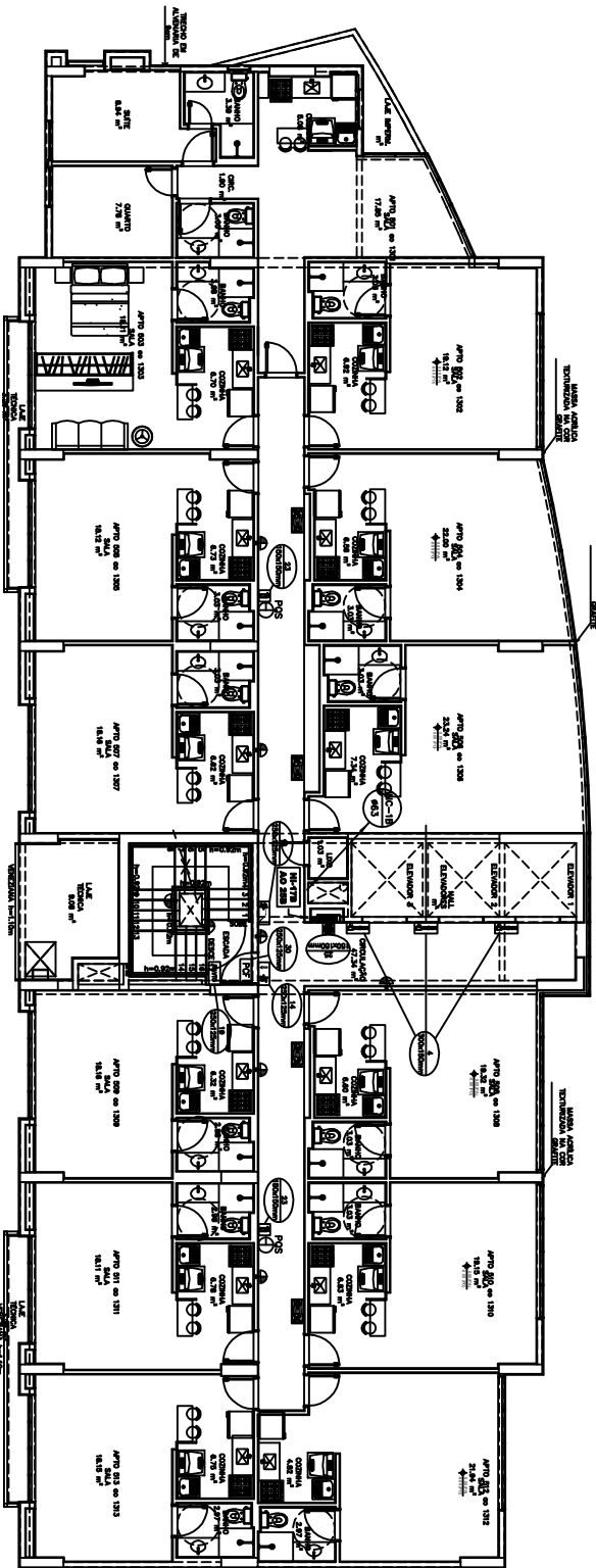
PLANTA BAIXA 5.º AO 13.º PAVIMENTO – BLOCO "B" RESIDENCIAL
