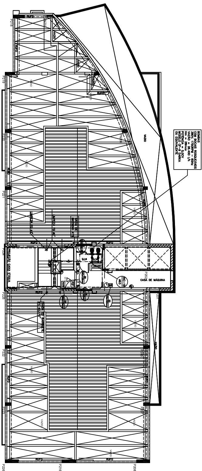
PLANTA BAIXA COBERTURA – BLOCO “B” RESIDENCIAL ESCALA 1:50
